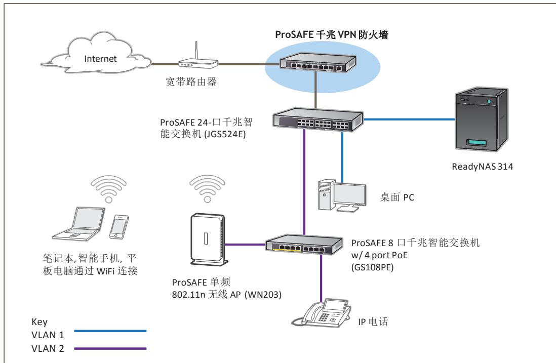
ProSAFE VPN 防火墙部署示意图
