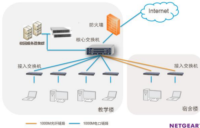
哈尔滨德强商务学院校园网络方案拓扑图
